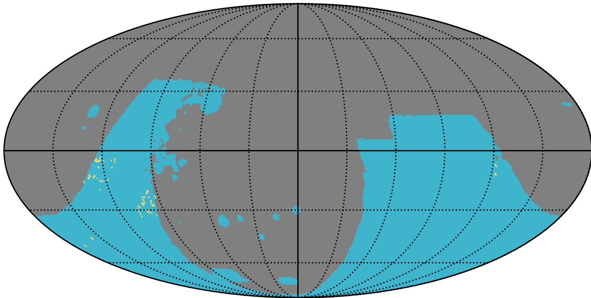
octo_v3.4_10yrs : GalplaneFootprintMetric_combined_map_Tau_5_0
