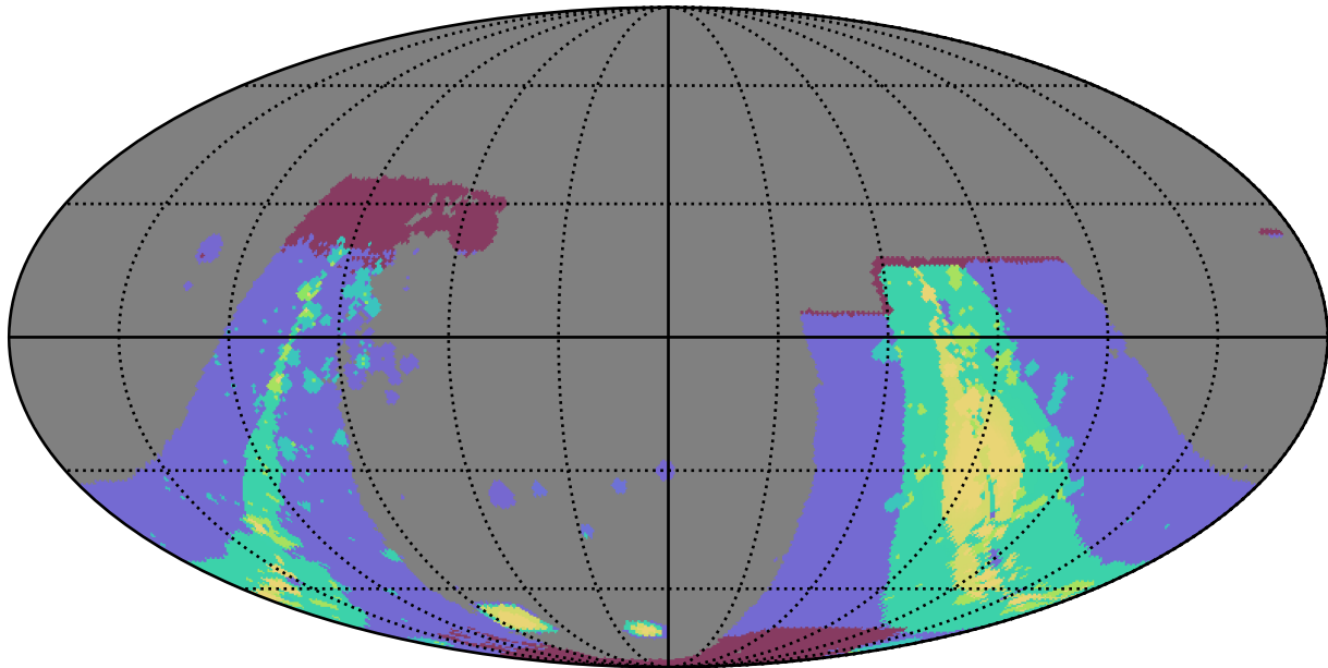
octo_v3.4_10yrs : GalplaneFootprintMetric_combined_map_Tau_46_5
