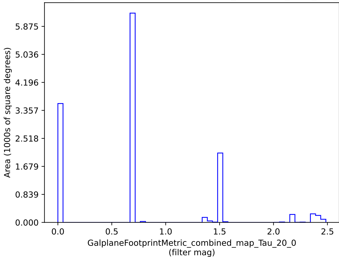
octo_v3.4_10yrs : GalplaneFootprintMetric_combined_map_Tau_20_0
