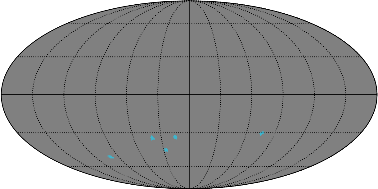
octo_v3.4_10yrs : GalplaneFootprintMetric_clementini_stellarpops_map_Tau_2_0
