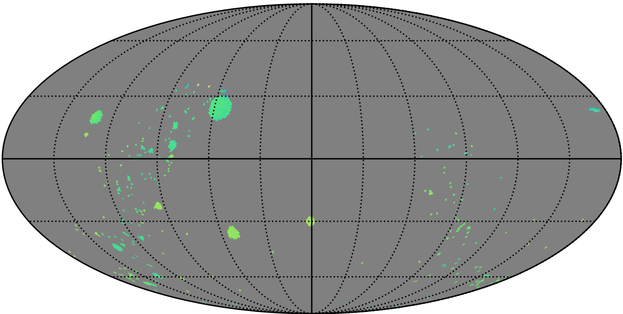
octo_v3.4_10yrs : GalPlaneVisitIntervalsTimescales_open_clusters_map_Tau_2_0
