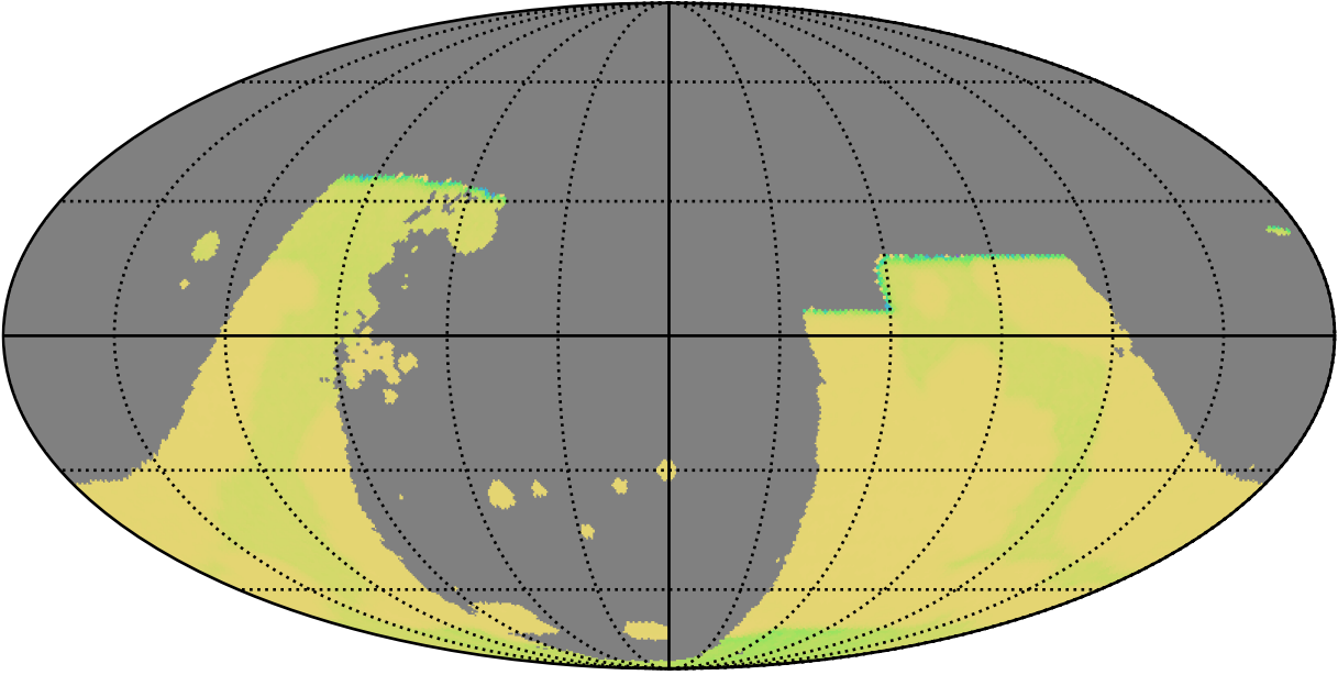
octo_v3.4_10yrs : GalPlaneVisitIntervalsTimescales_combined_map_Tau_73_0
