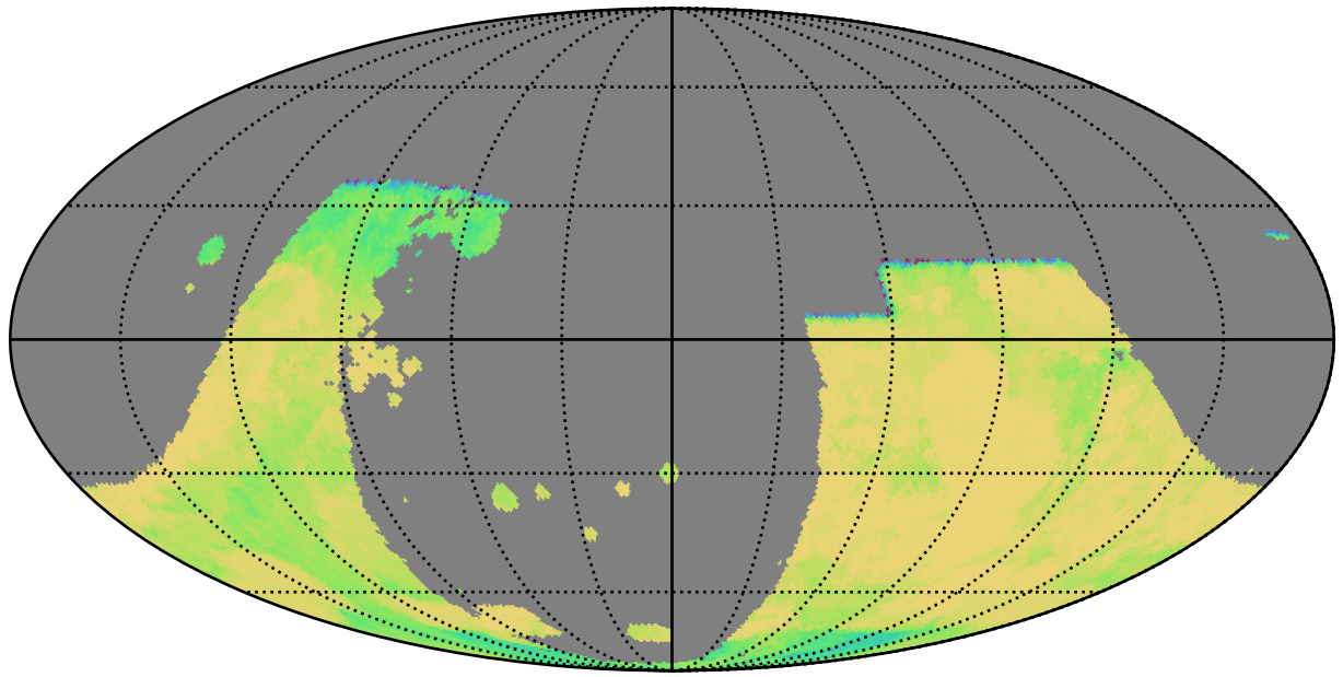
octo_v3.4_10yrs : GalPlaneSeasonGapsTimescales_combined_map_Tau_232_5
