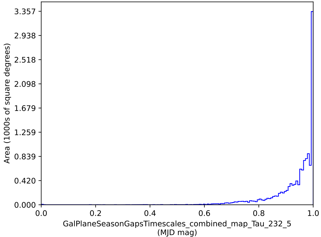
octo_v3.4_10yrs : GalPlaneSeasonGapsTimescales_combined_map_Tau_232_5
