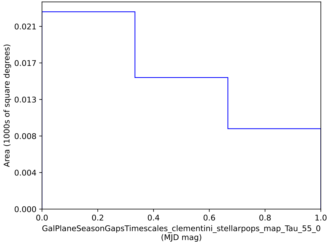
octo_v3.4_10yrs : GalPlaneSeasonGapsTimescales_clementini_stellarpops_map_Tau_55_0
