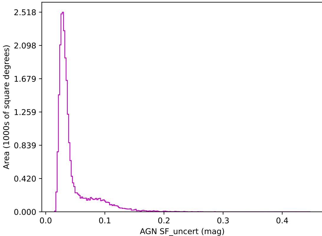
octo_v3.4_10yrs z band: AGN SF_uncert
