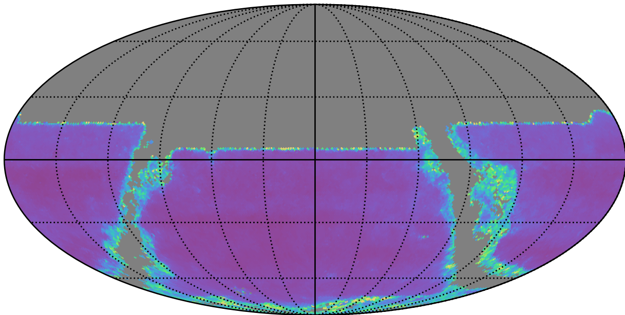
octo_v3.4_10yrs y band: AGN SF_uncert
