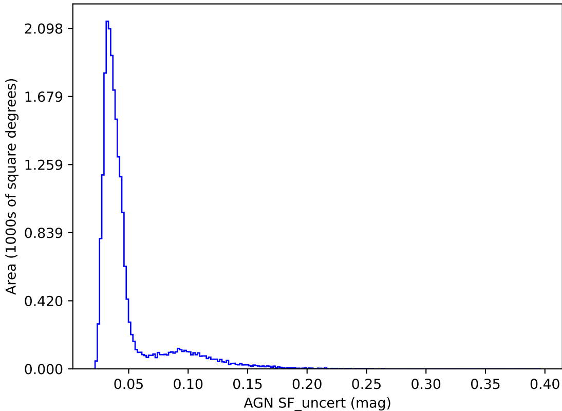
octo_v3.4_10yrs y band: AGN SF_uncert
