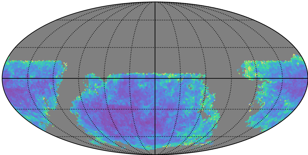
octo_v3.4_10yrs u band: AGN SF_uncert
