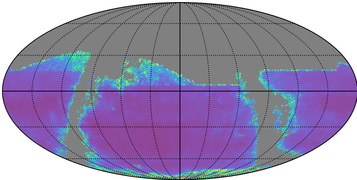
octo_v3.4_10yrs r band: AGN SF_uncert
