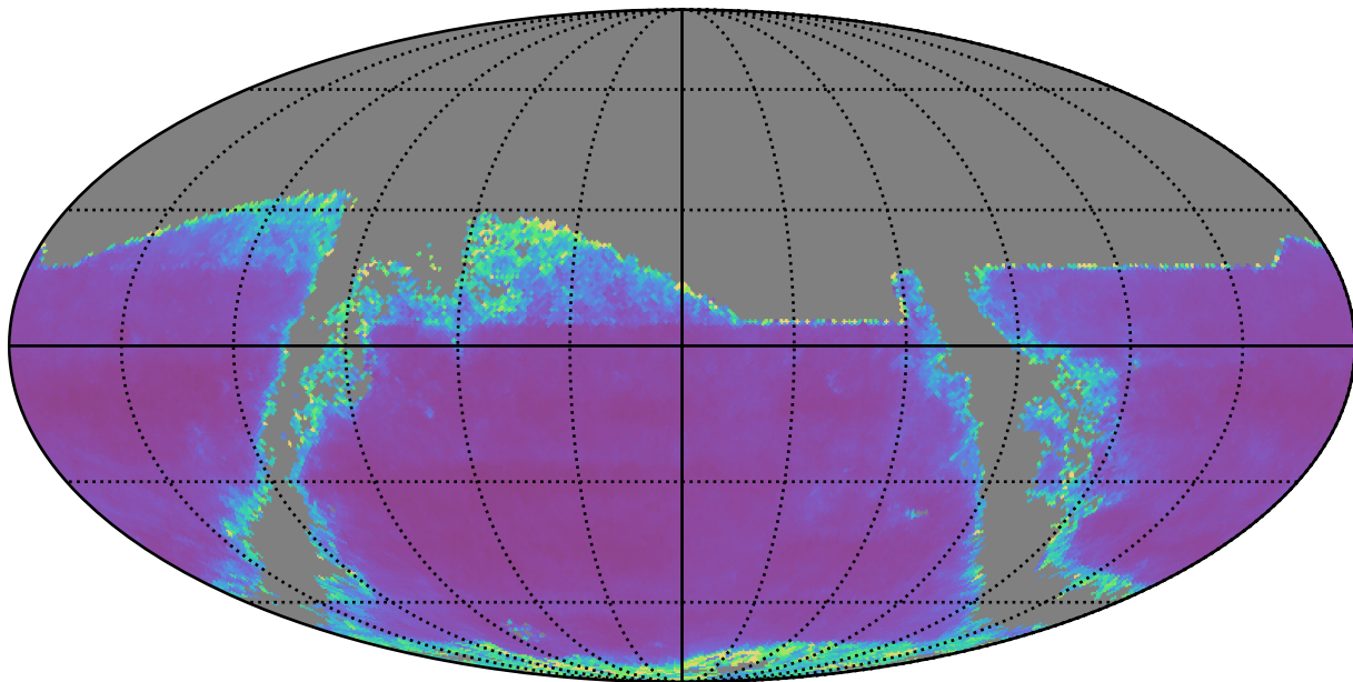
octo_v3.4_10yrs i band: AGN SF_uncert
