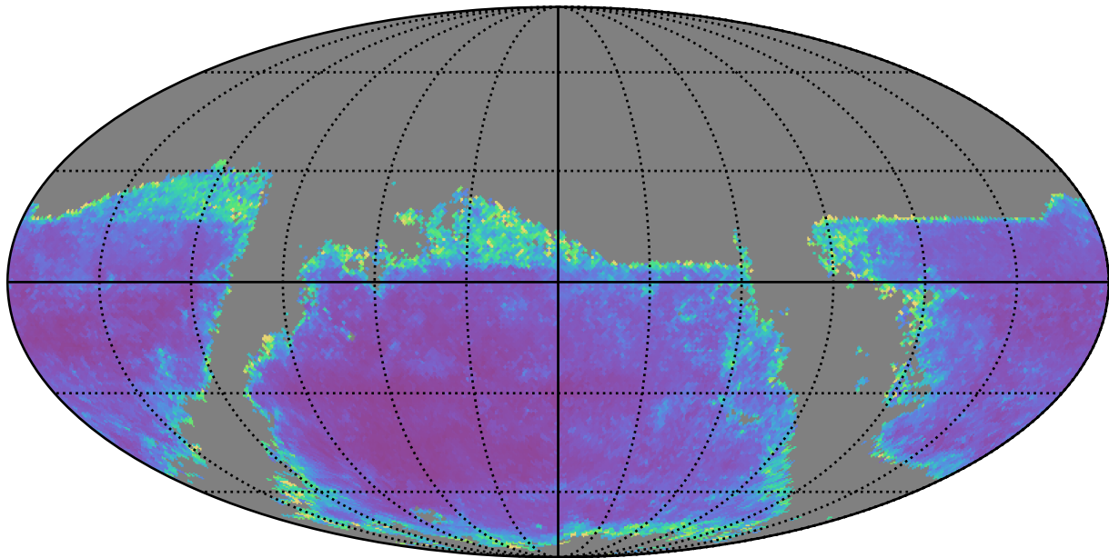
octo_v3.4_10yrs g band: AGN SF_uncert
