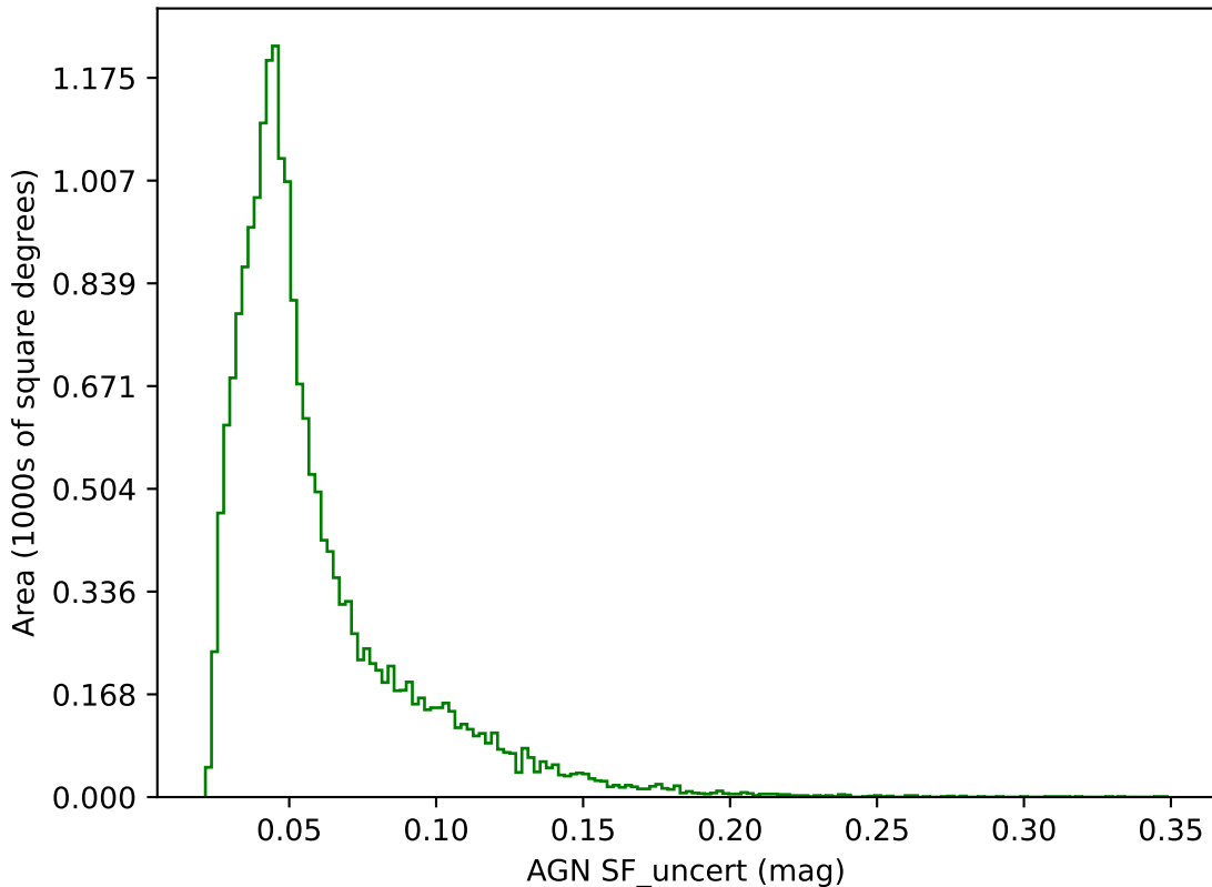
octo_v3.4_10yrs g band: AGN SF_uncert
