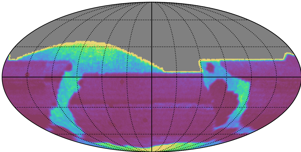
octo_v3.4_10yrs : properMotion
