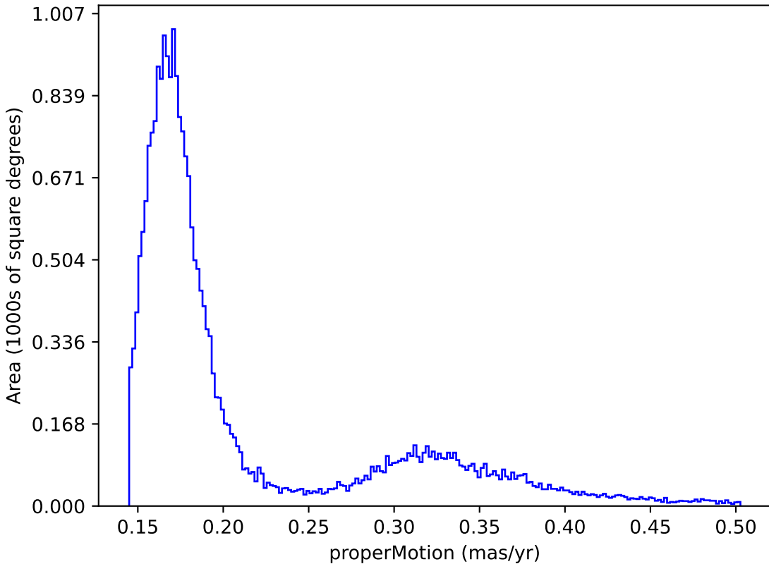
octo_v3.4_10yrs : properMotion
