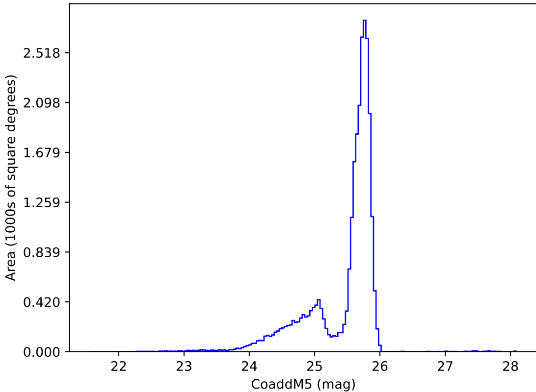
octo_v3.4_10yrs z: CoaddM5
