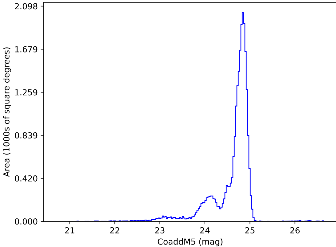
octo_v3.4_10yrs y: CoaddM5
