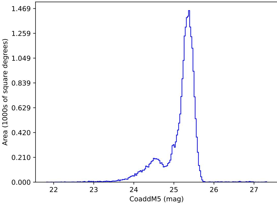
octo_v3.4_10yrs u: CoaddM5
