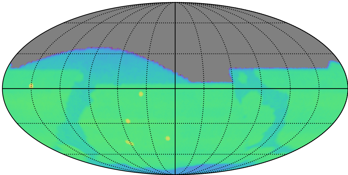
octo_v3.4_10yrs r: CoaddM5
