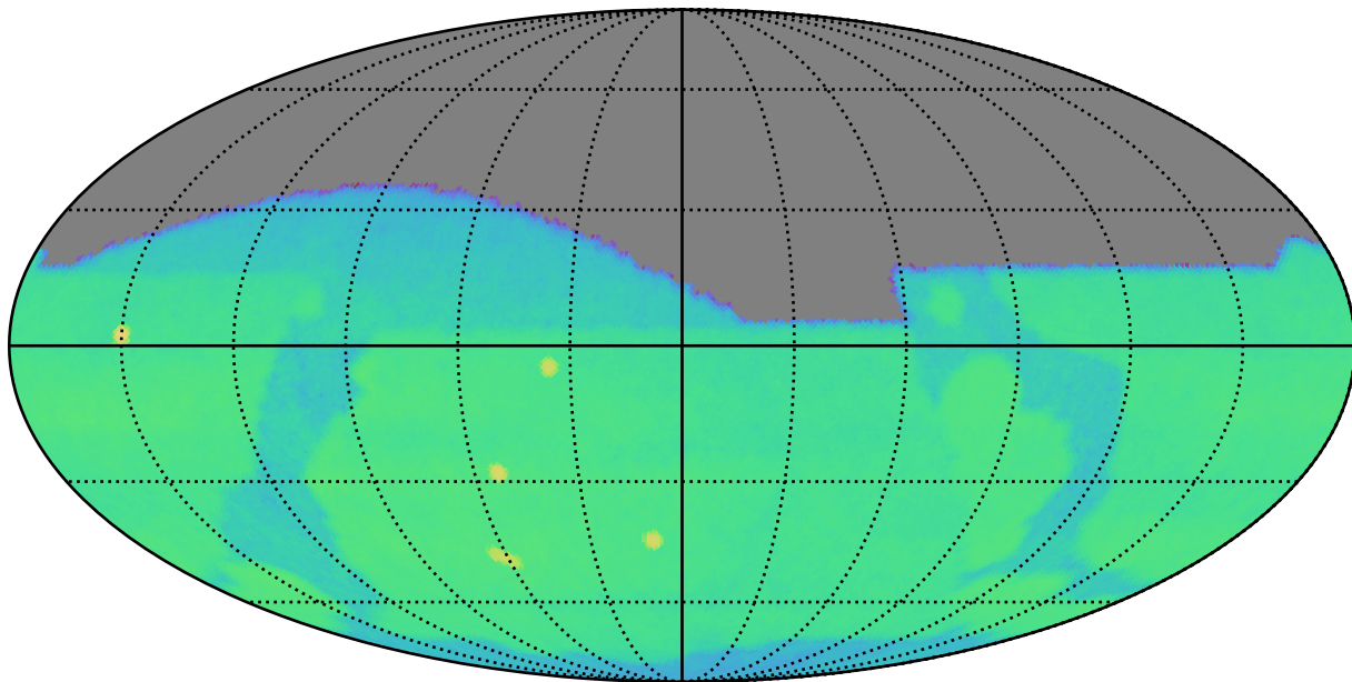
octo_v3.4_10yrs g: CoaddM5
