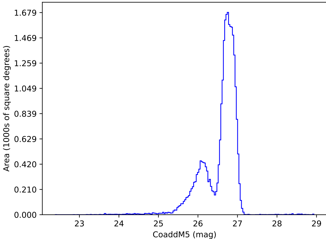
octo_v3.4_10yrs g: CoaddM5
