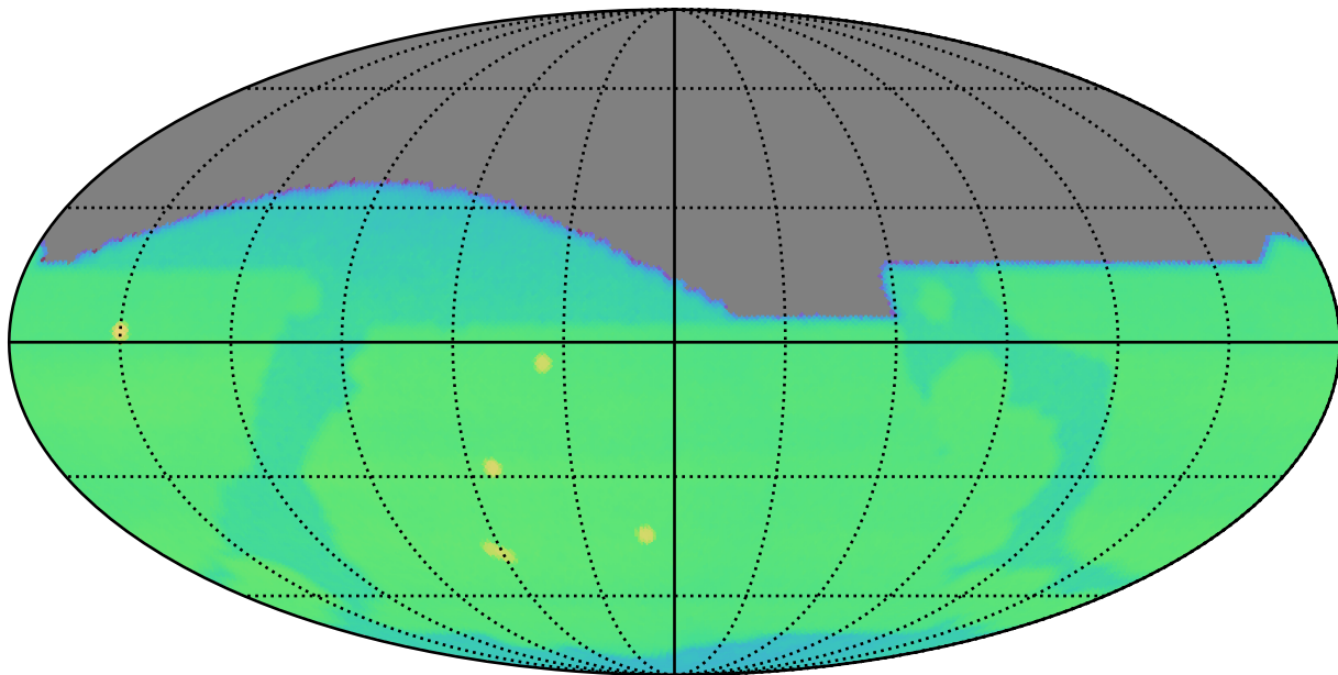
octo_v3.4_10yrs : CoaddM5
