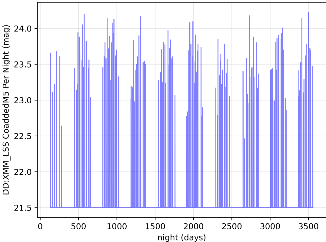
octo_v3.4_10yrs y band: DD:XMM_LSS CoaddedM5 Per Night
