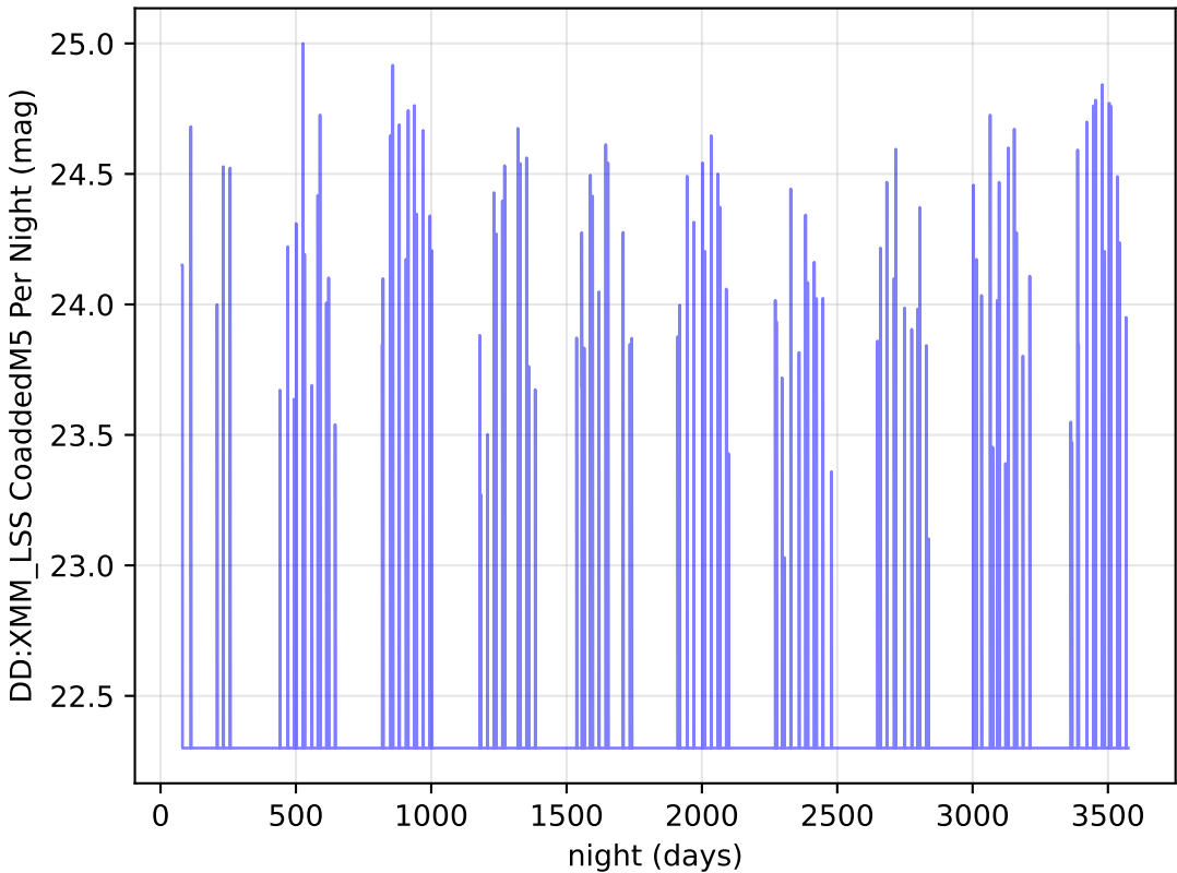
octo_v3.4_10yrs u band: DD:XMM_LSS CoaddedM5 Per Night
