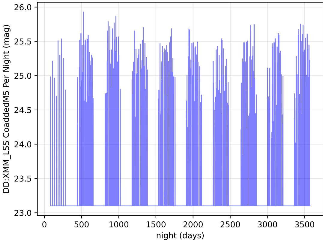
octo_v3.4_10yrs i band: DD:XMM_LSS CoaddedM5 Per Night
