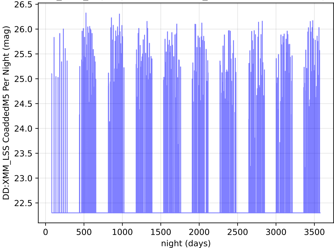
octo_v3.4_10yrs g band: DD:XMM_LSS CoaddedM5 Per Night
