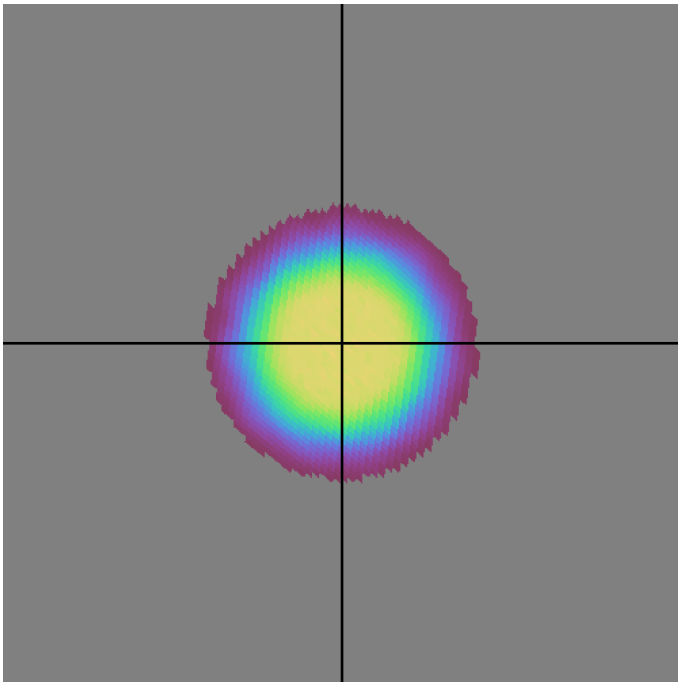
octo_v3.4_10yrs all bands: DD:ELAISS1 NVisits
