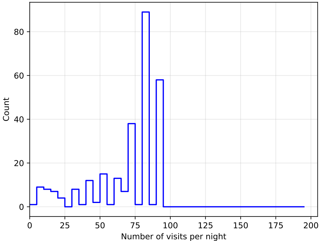
octo_v3.4_10yrs all bands: DD:ELAISS1 NVisitsPerNight
