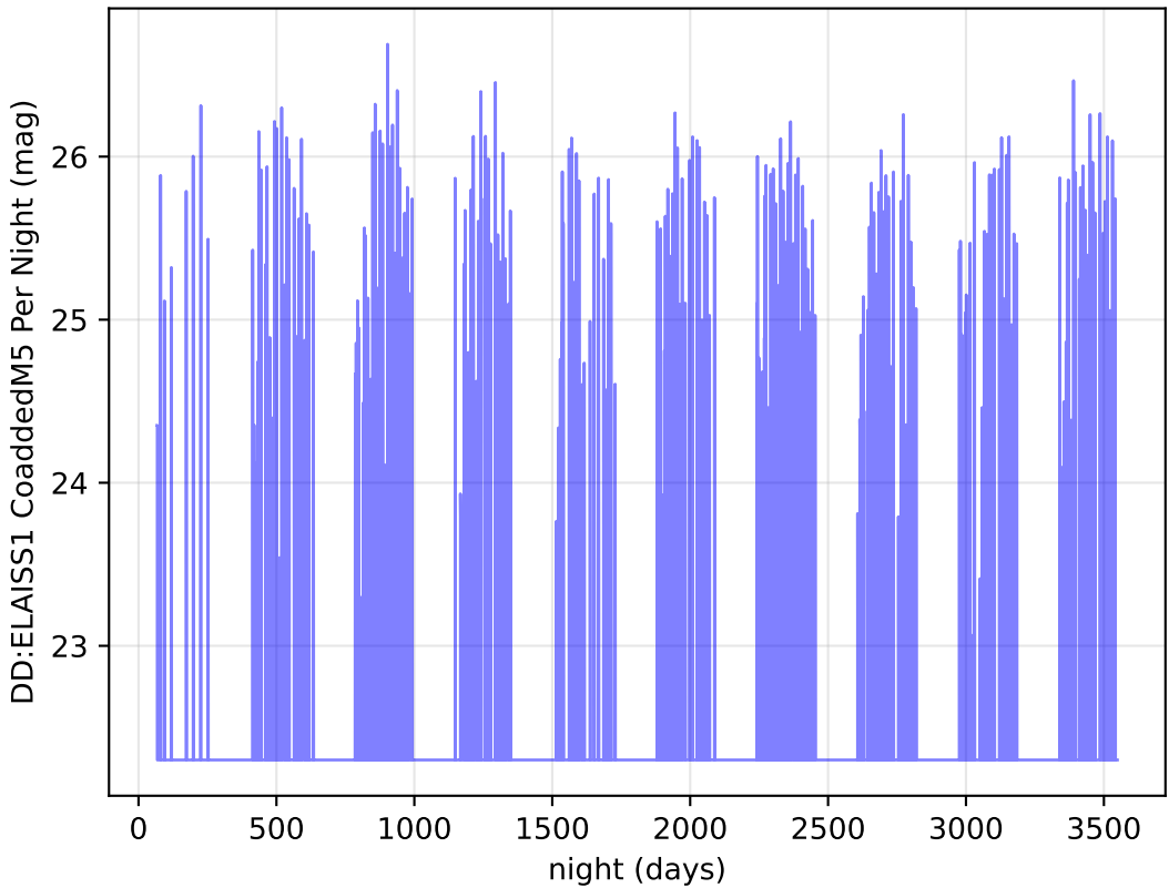
octo_v3.4_10yrs g band: DD:ELAISS1 CoaddedM5 Per Night
