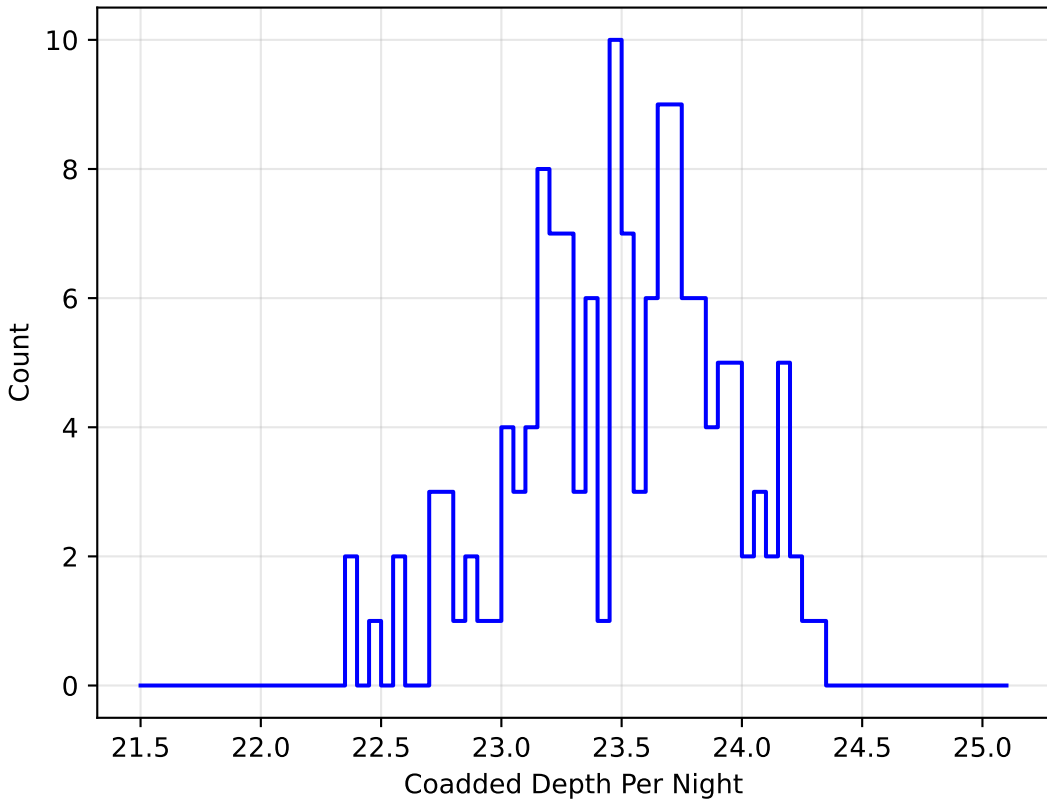
octo_v3.4_10yrs y band: DD:ELAISS1 CoaddM5PerNight
