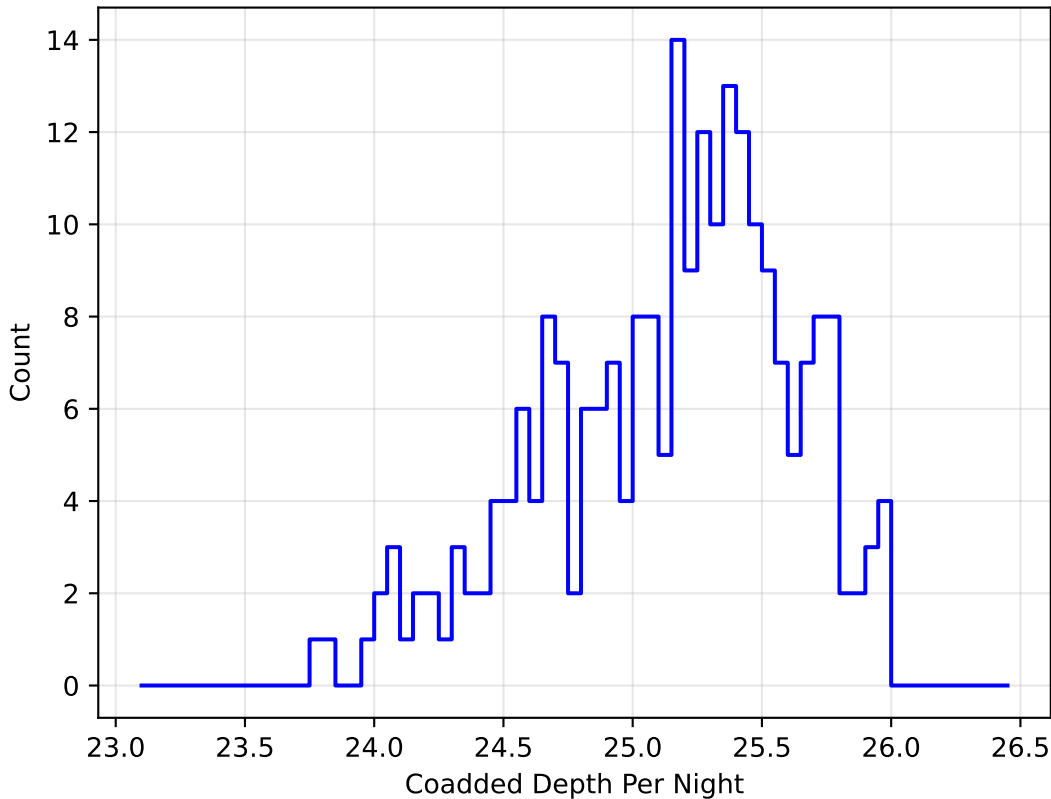
octo_v3.4_10yrs i band: DD:ELAISS1 CoaddM5PerNight
