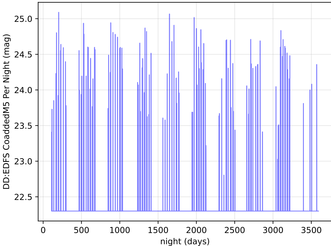
octo_v3.4_10yrs u band: DD:EDFS CoaddedM5 Per Night
