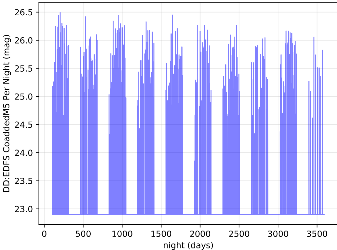
octo_v3.4_10yrs r band: DD:EDFS CoaddedM5 Per Night
