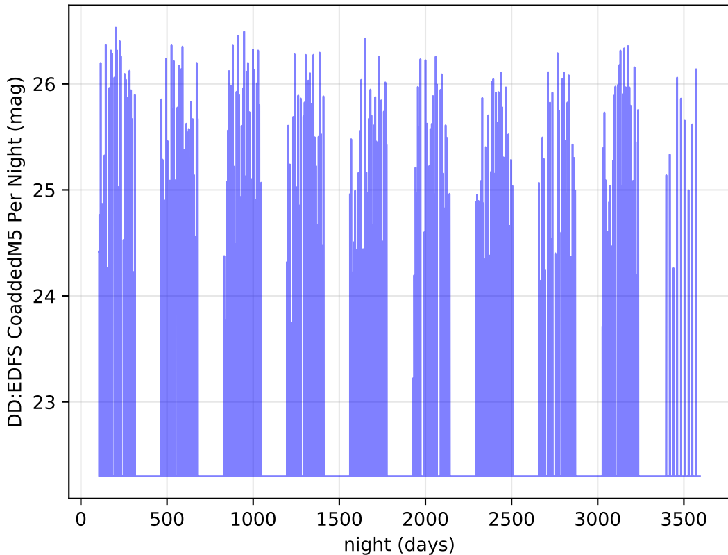
octo_v3.4_10yrs g band: DD:EDFS CoaddedM5 Per Night
