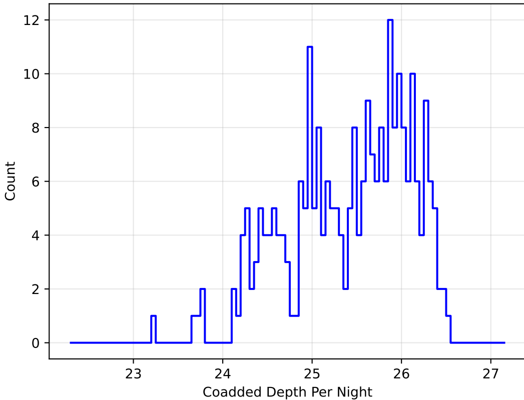
octo_v3.4_10yrs g band: DD:EDFS CoaddM5PerNight
