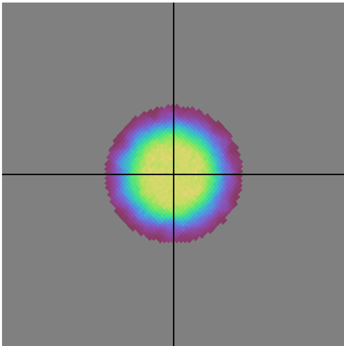
octo_v3.4_10yrs g band: DD:ECDFS NVisits
