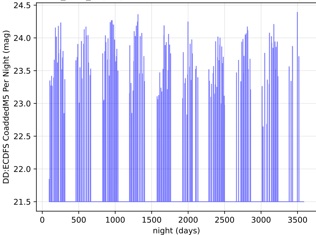
octo_v3.4_10yrs y band: DD:ECDFS CoaddedM5 Per Night
