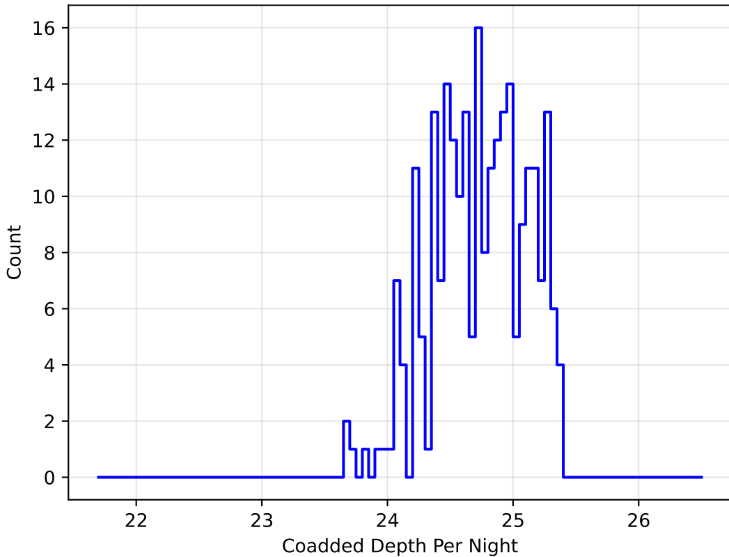
octo_v3.4_10yrs z band: DD:ECDFS CoaddM5PerNight
