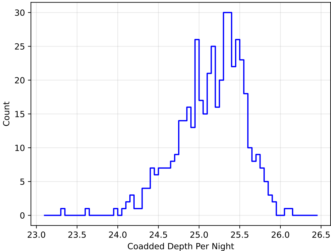
octo_v3.4_10yrs i band: DD:COSMOS CoaddM5PerNight
