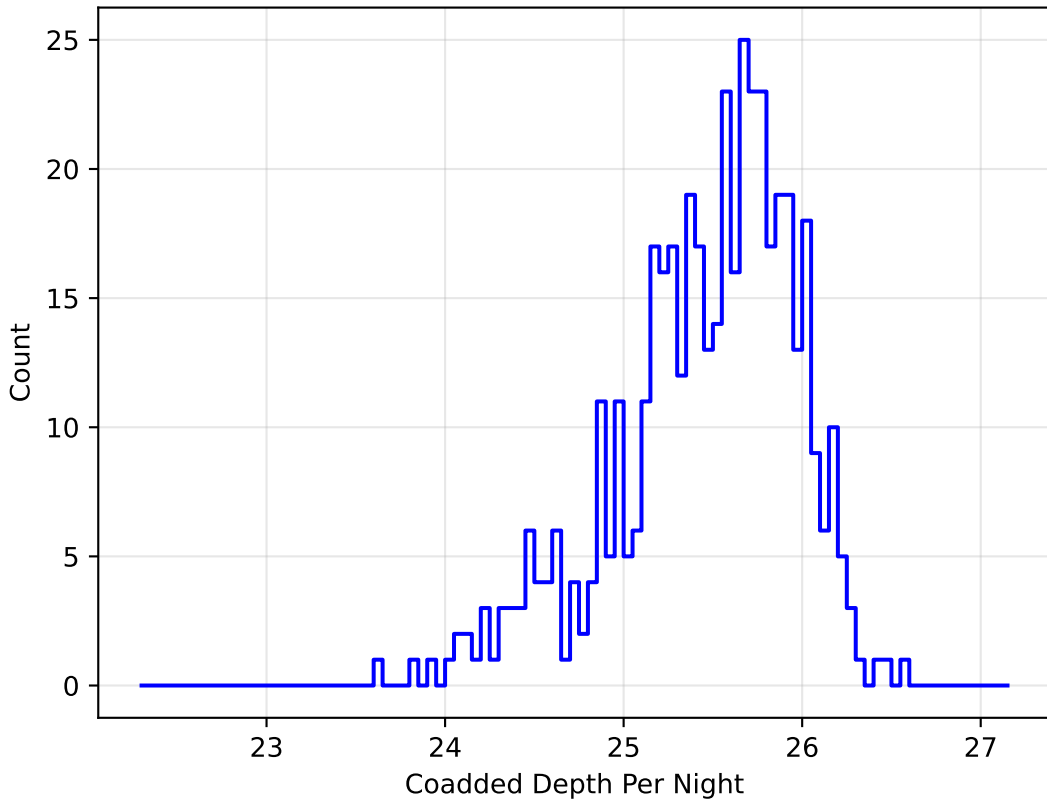
octo_v3.4_10yrs g band: DD:COSMOS CoaddM5PerNight
