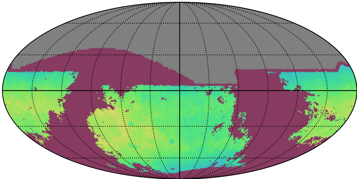
noroll_v3.4_10yrs i: NgalScale
