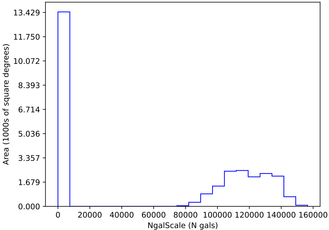
noroll_v3.4_10yrs i: NgalScale
