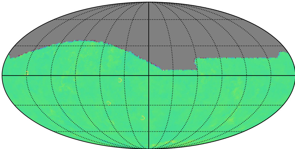
noroll_v3.4_10yrs z: Kuiper rotTelPos
