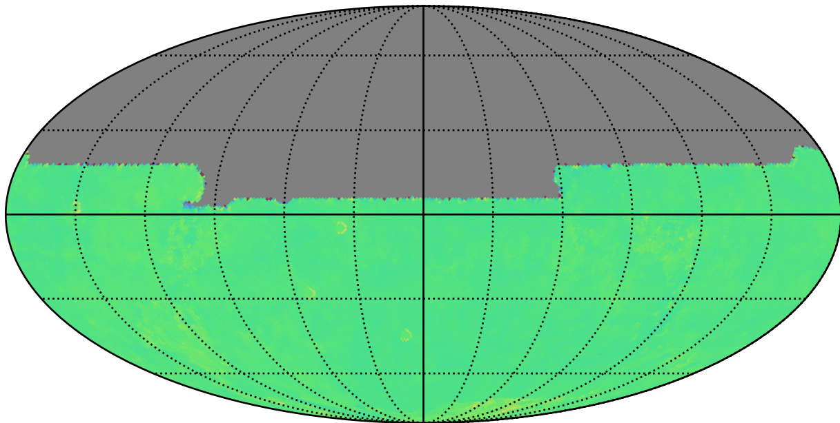
noroll_v3.4_10yrs y: Kuiper rotTelPos
