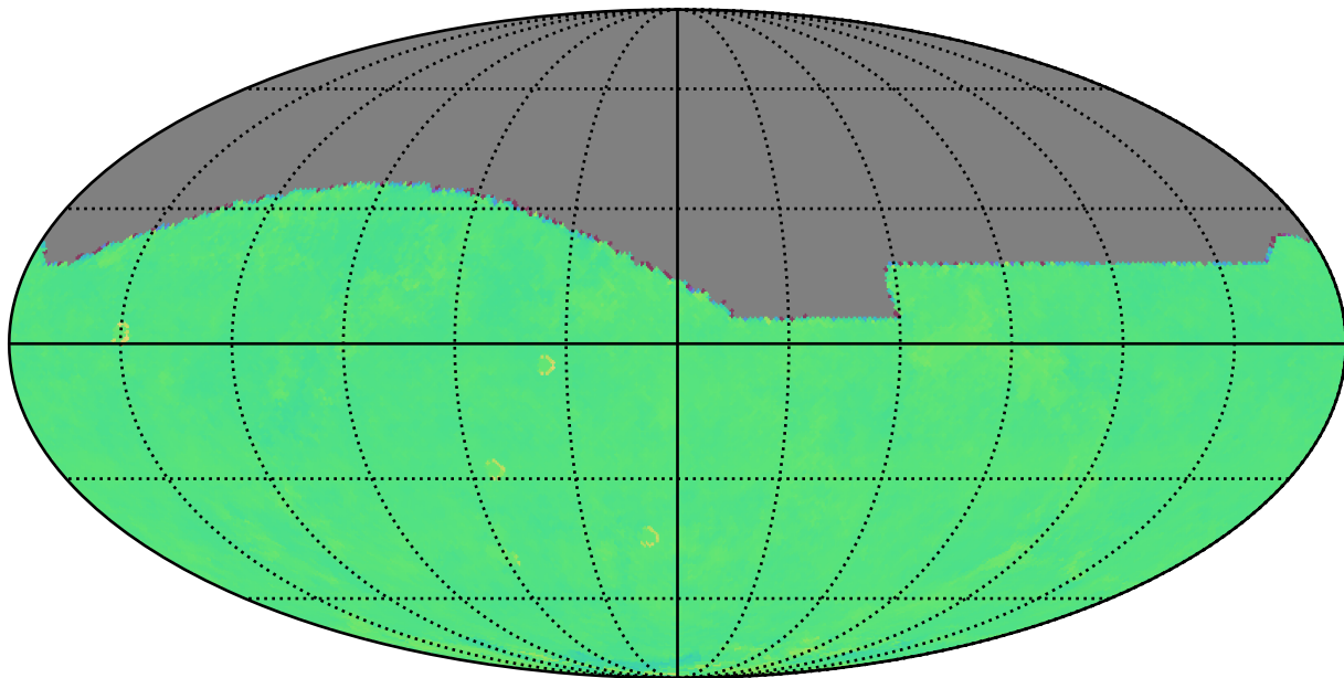
noroll_v3.4_10yrs r: Kuiper rotTelPos
