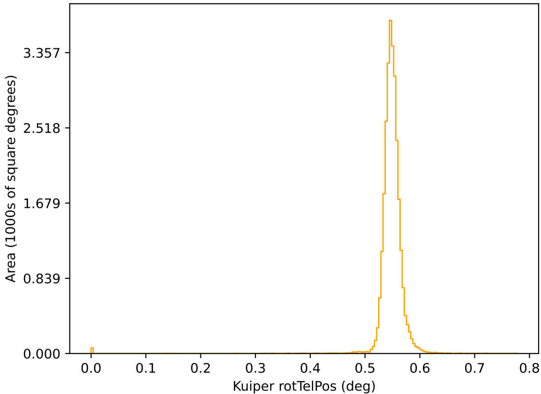
noroll_v3.4_10yrs r: Kuiper rotTelPos
